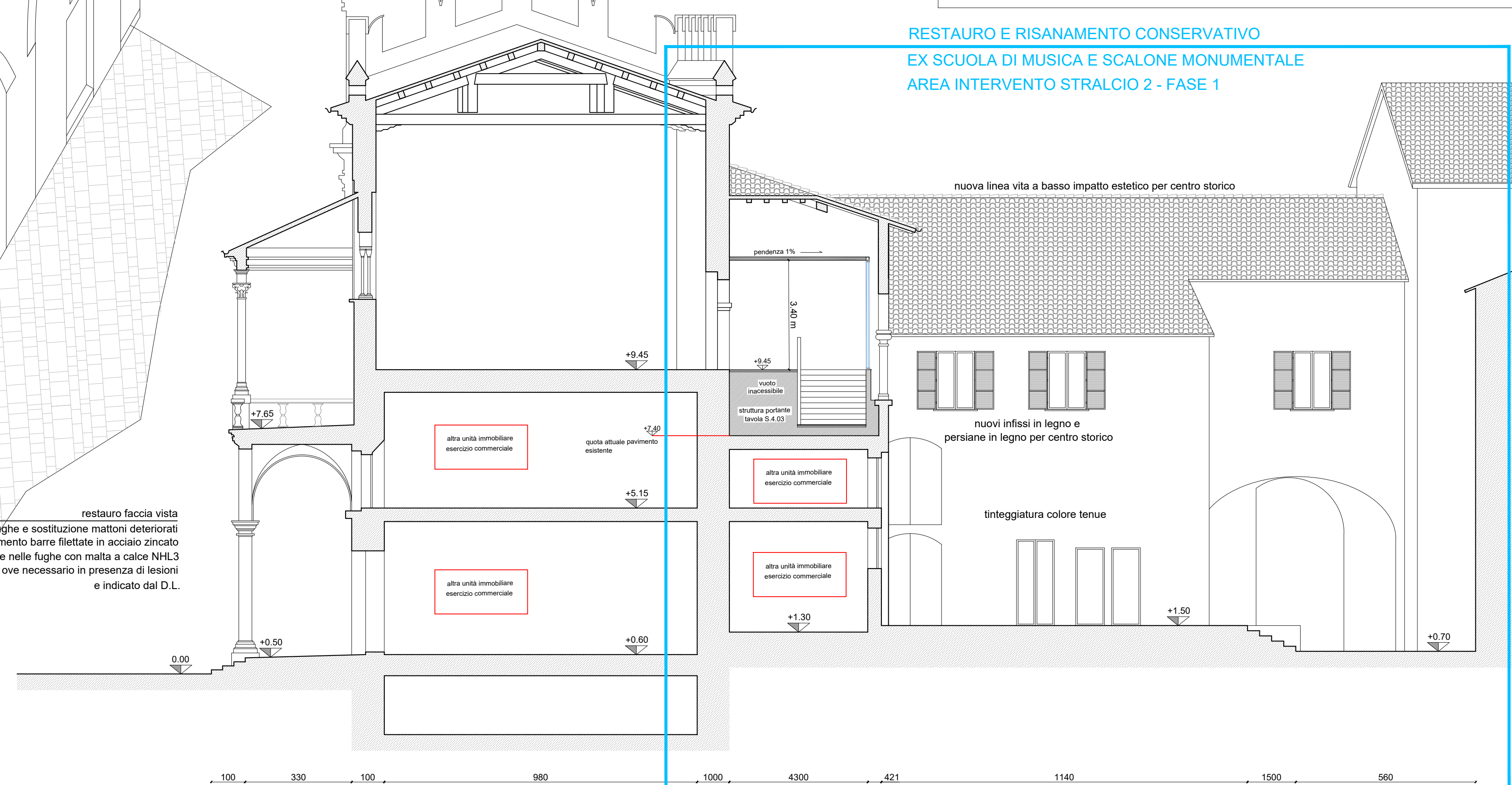
SEZIONE SCALONE STORICO DI INGRESSO
