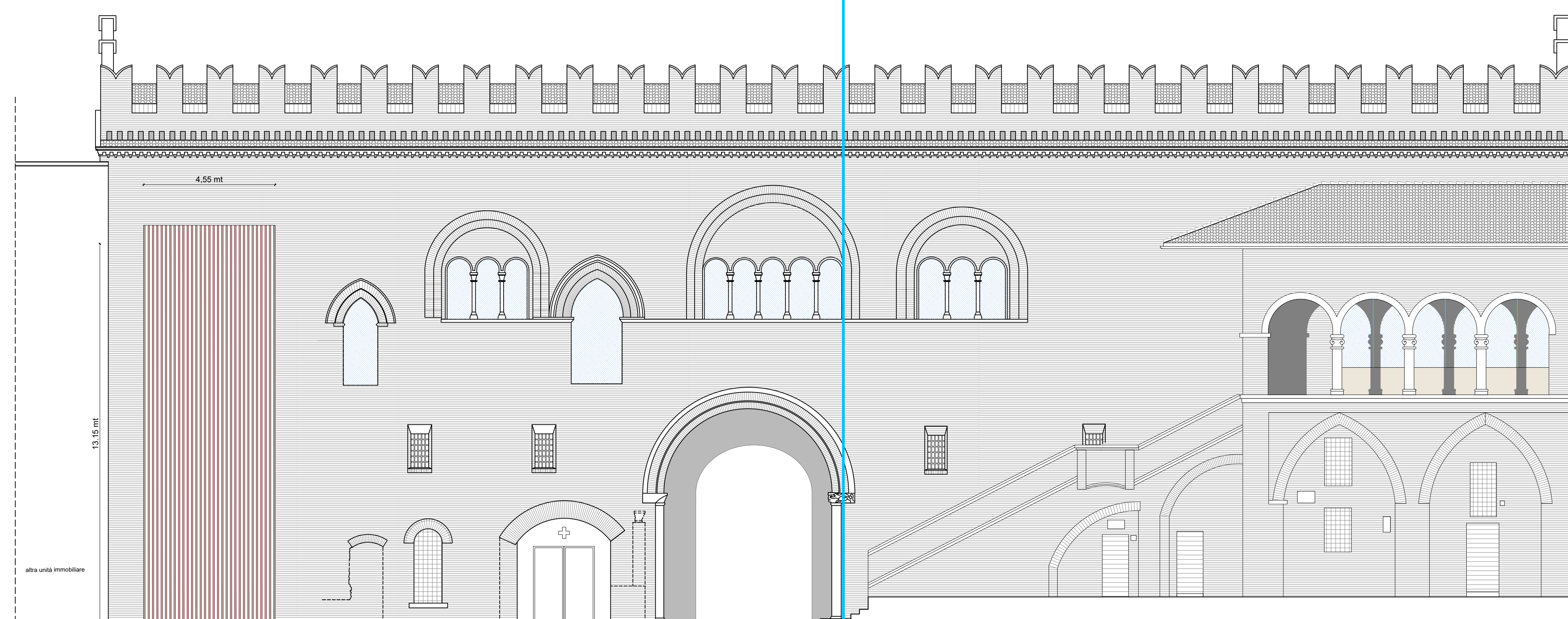
PROSPETTO - PALAZZO DEL PODESTÀ PIAZZA MARTIRI DELLE LIBERTÀ
