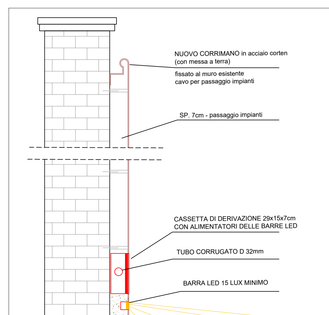
PARTICOLARE SEZIONE DEL CORRIMANO SCALONE MONUMENTALE E VIA D'ESODO US
